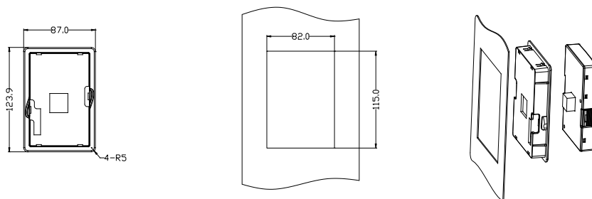
Gniazdo montażowe (0.75~500kW) (opcjonalnie)
