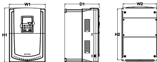
Montaż ścienny przemienników 400V 18.5-30kW
