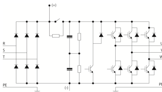
Rys. 3-1 Schemat obwodu mocy ( \leq 30\text{kW} )
