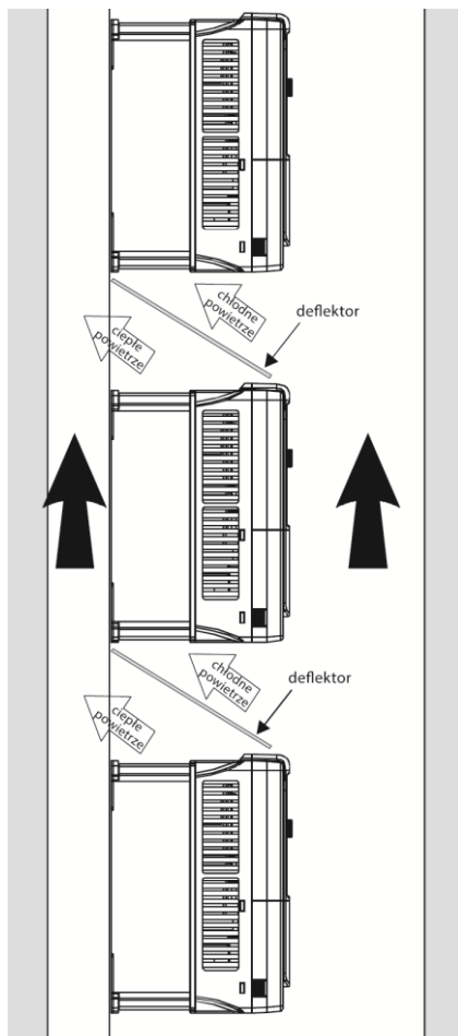
Rys. 4-5 Rozmieszczenie pionowe
