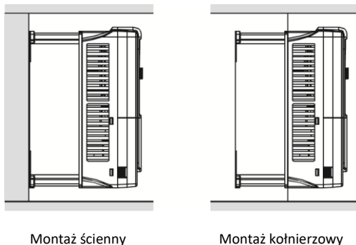
Rys. 4-2 Sposób instalacji
