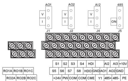
Rys. 4-21 Terminal obwodu sterowania (0.75~15kW)
