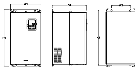
Montaż ścienny przemienników 400V 37-110kW
