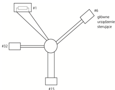
Rys. 10-3 Topologia „gwiazdy”
