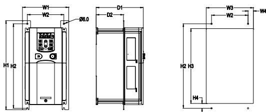
Montaż kołnierzowy przemienników 400V 0.75-15kW
