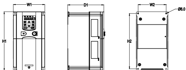
Montaż ścienny przemienników 400V 1.5-15kW
