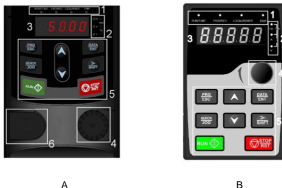
Rys. 5-1 Panel sterowania
