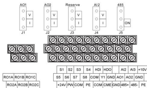
Rys. 4-22 Terminal obwodu sterowania (18.5~500kW)
