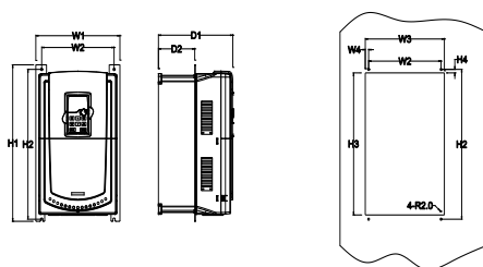
Montaż kołnierzowy przemienników 400V 18.5-30kW
